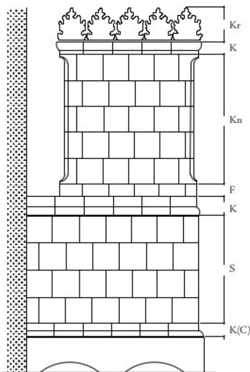
1 Marijos Dąbrowskos koklių tipų schema: karūniniai kokliai (Kr); karniziniai (K, K(C)) [karniziniai-cokoliniai vidiniai]; kampiniai kairysis/dešinysis; friziniai (F) [vidiniai; kampiniai kairysis/dešinysis]; sieniniai (S) [vidiniai; kampiniai kairysis/dešinysis]; kampiniai nišiniai (Kn)
