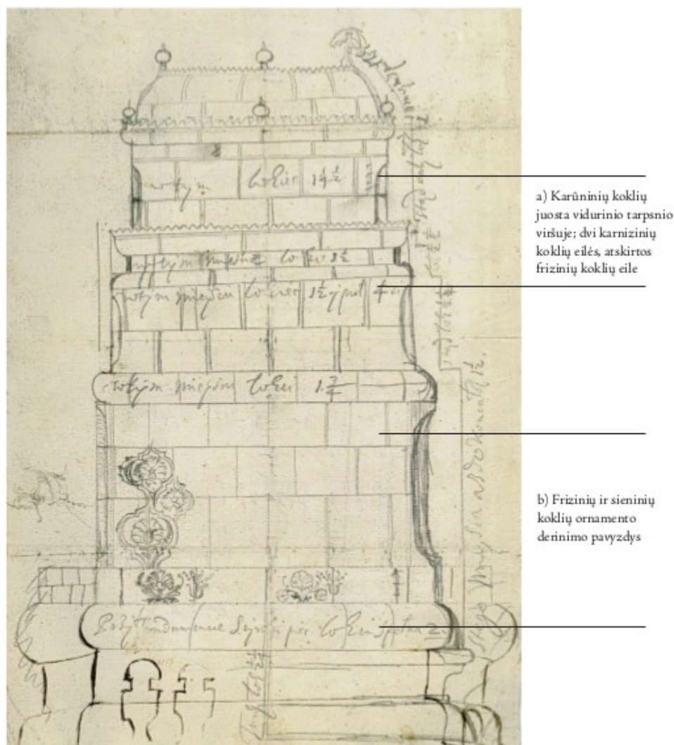
16 Krosnies brėžinys iš Radvilų archyvo. XVII a. vid.
